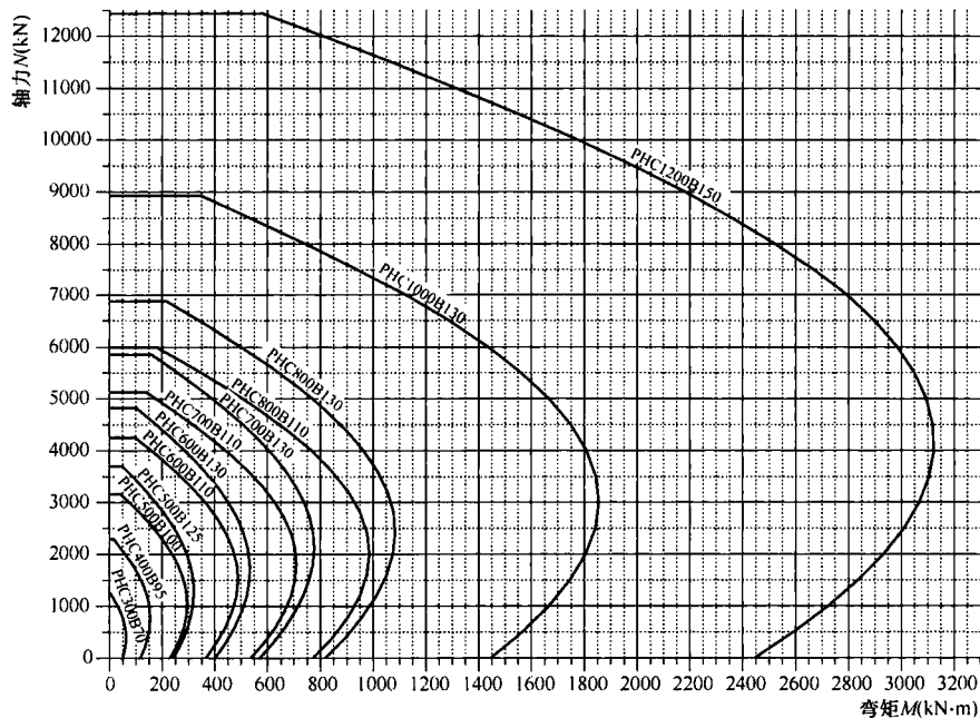
图 B.0.3 PHC 管桩 B 型偏心受压 N-M 曲线
