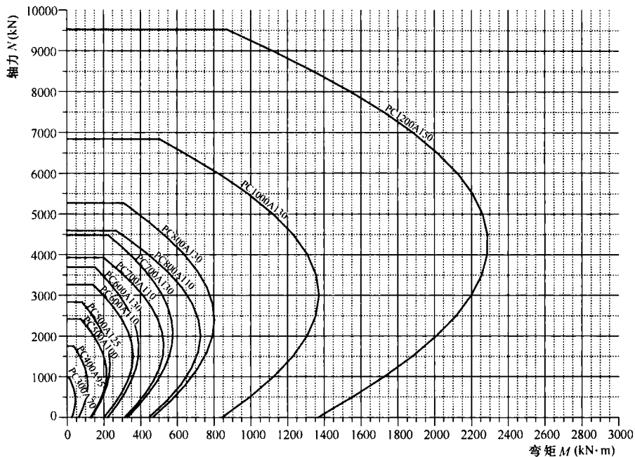
图 B.0.5 PC 管桩 A 型偏心受压 N-M 曲线
