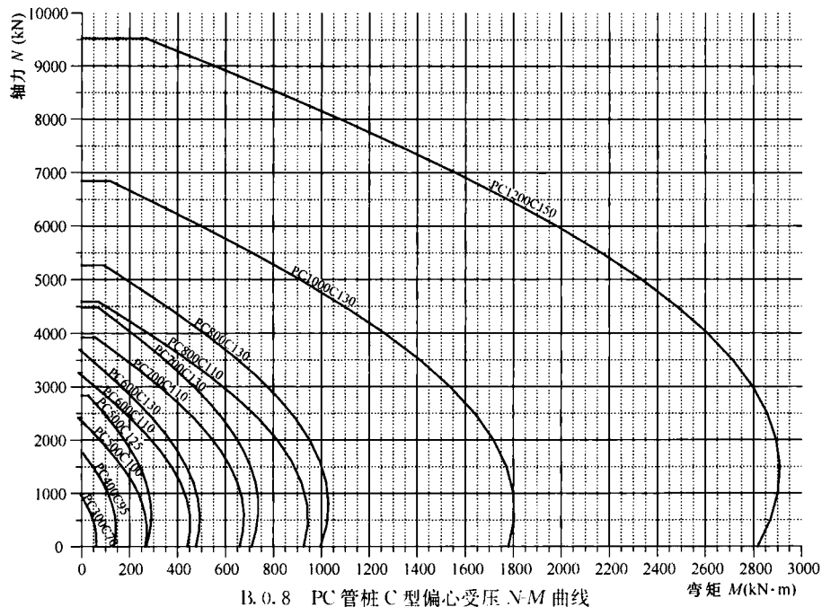
B.0.8 PC管桩C型偏心受压 N-M 曲线(图 B.0.8)。
