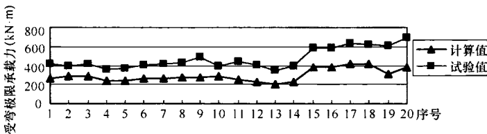
(c) 式 (8) 计算值与试验值对比
