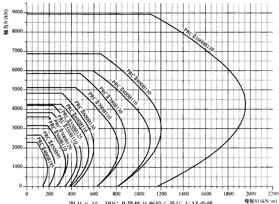
图 B. 0. 16 PRC-Ⅱ管桩B型偏心受压 N-M 曲线
