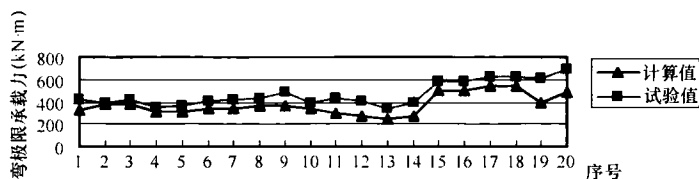
(a) 式 (2) 计算值与试验值对比
