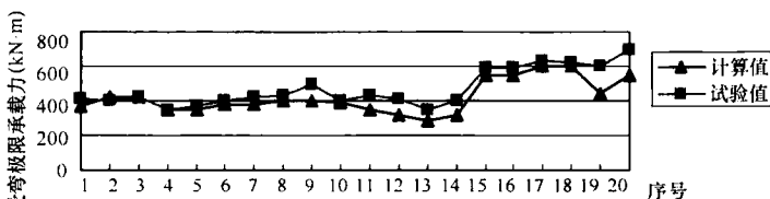
(b) 式 (5) 计算值与试验值对比
