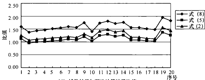
(d) 试验结果与理论计算结果比值
